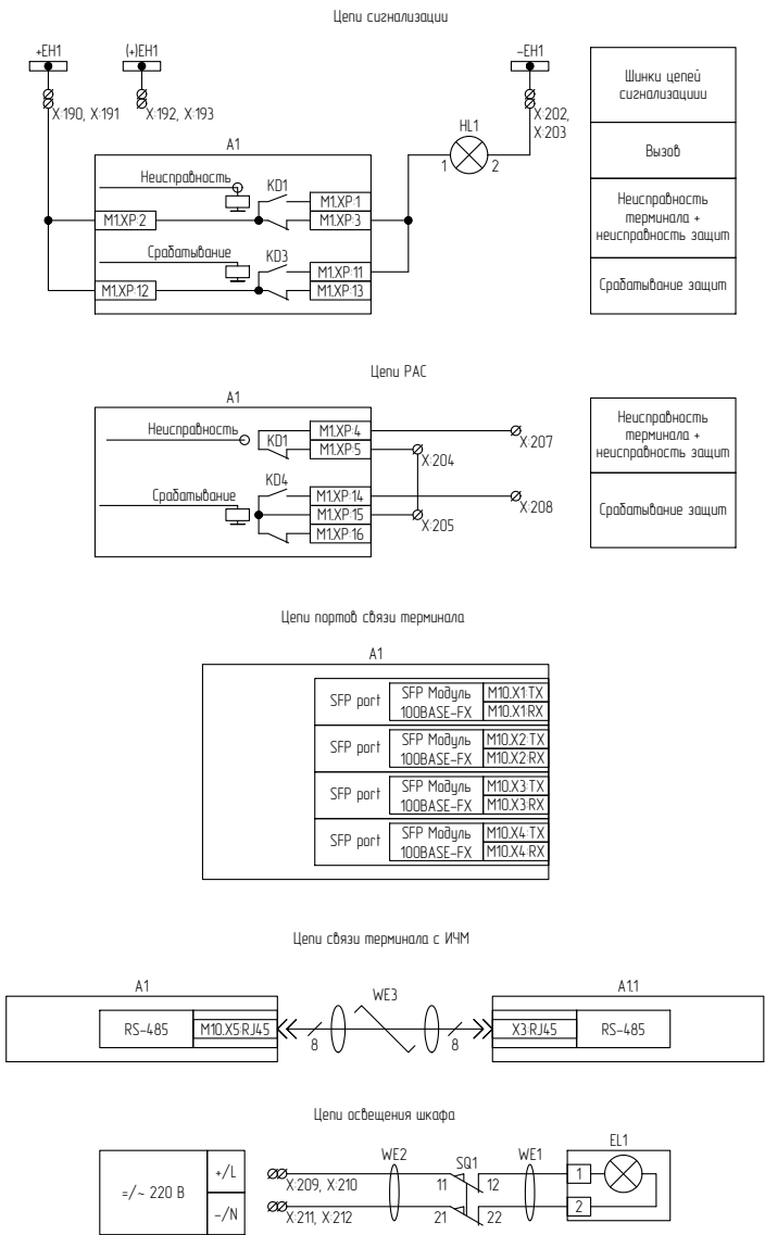
Рисунок Г.5 – Схема электрическая принципиальная (часть 5)
